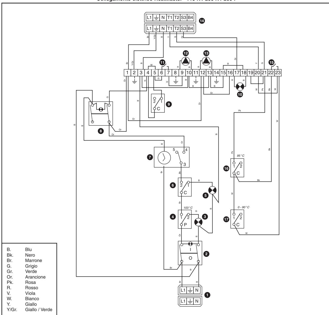
Collegamento elettrico HeatMaster® 115 N / 200 N / 200 F
